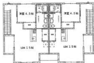
2階平面図
