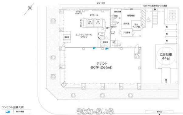
1階(テナント)平面図
